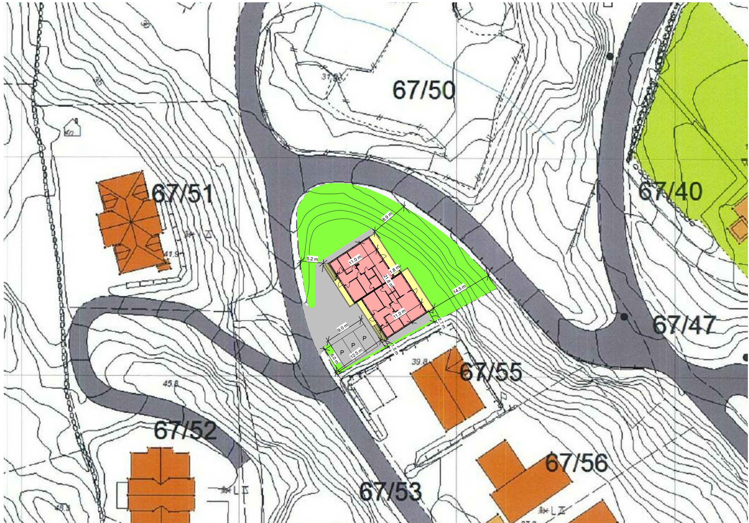
Situasjonskart 1 : 500
